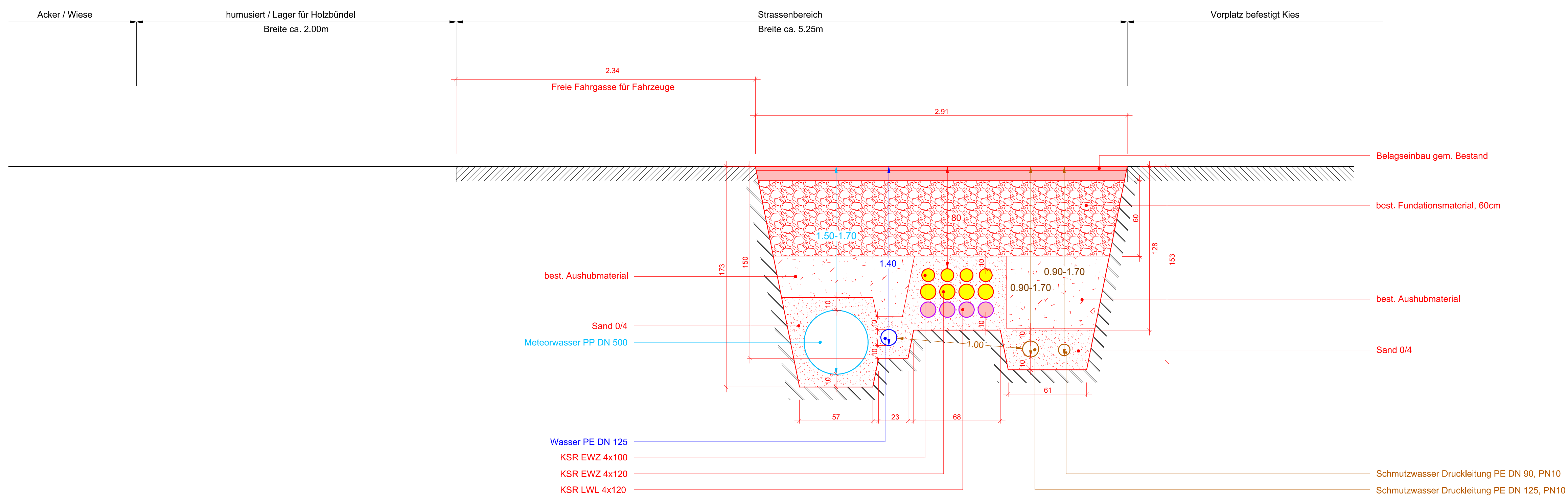
Grabenprofil 2 1. Etappe 1:20
