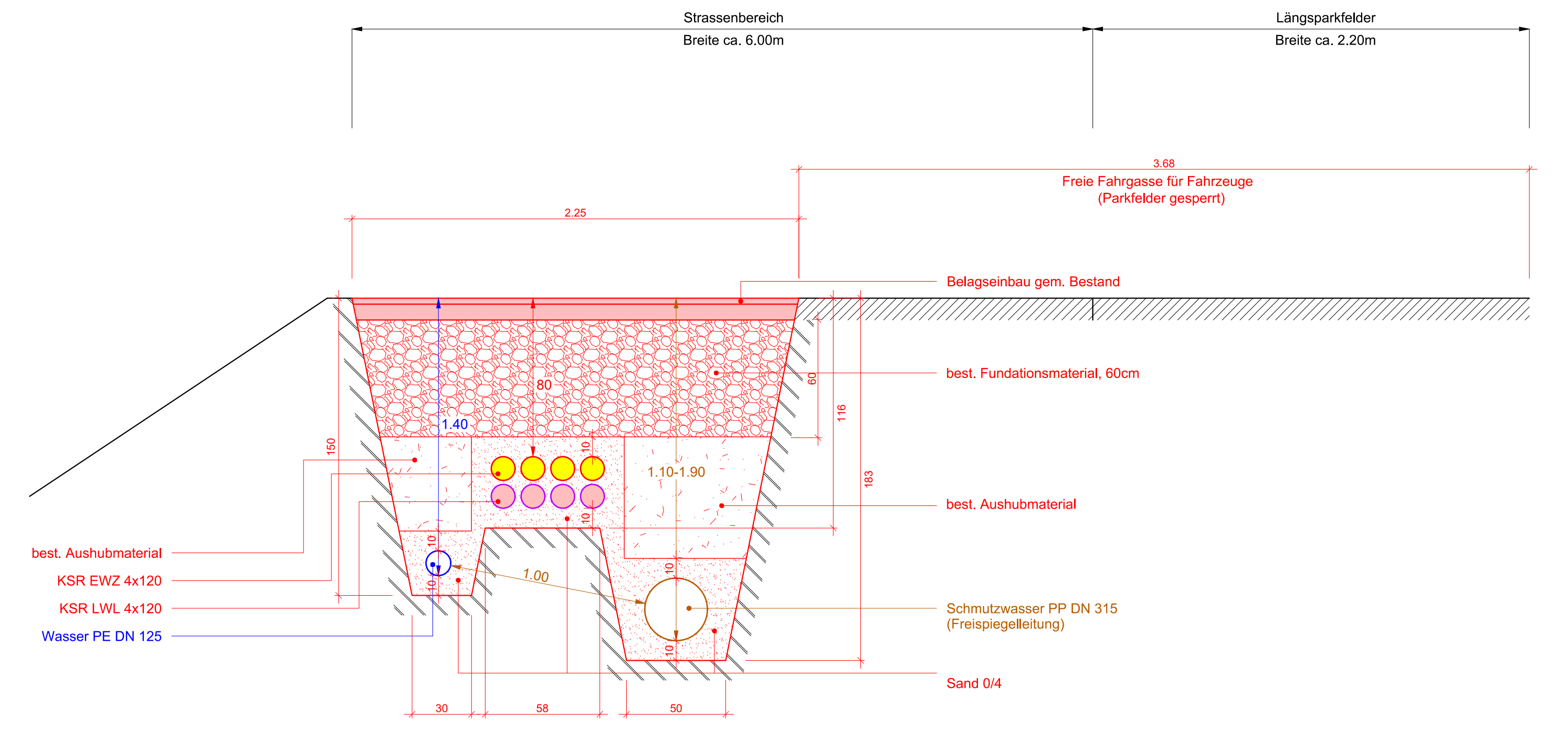
Grabenprofil 4 1. Etappe 1:20
