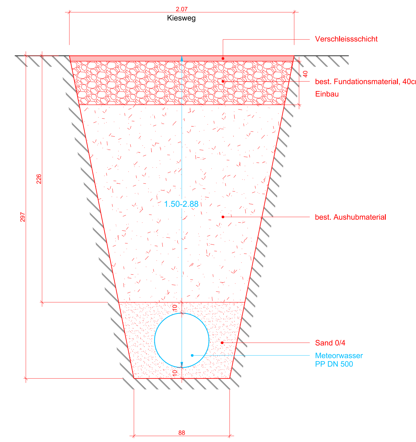
Grabenprofil 3 1. Etappe 1:20
