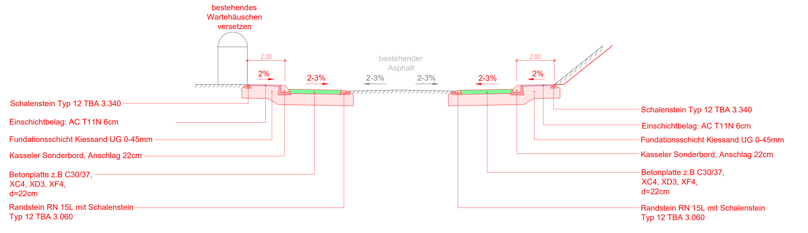
Schnitt 1-1 1:100
